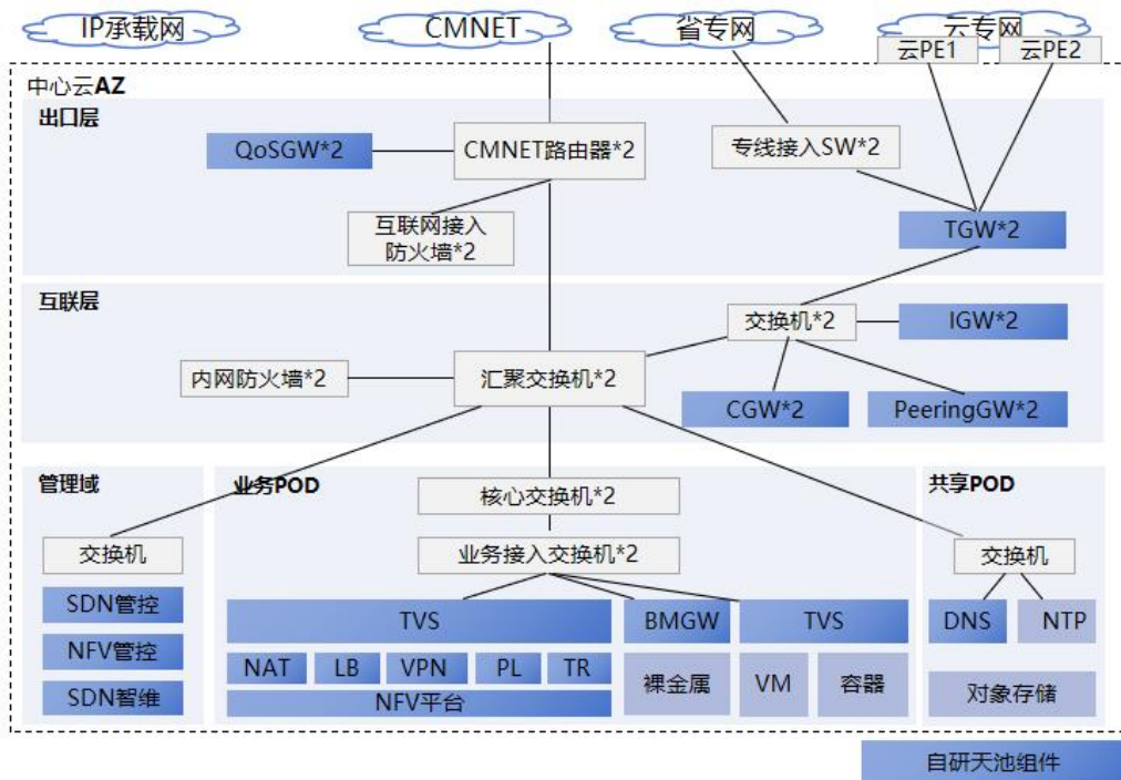
图 11 云内 SDN 网络架构示意图
